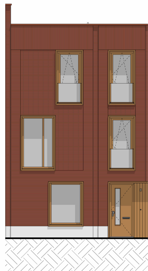
voorgevel 1 : 100
